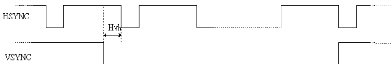
(D) HSYNC, VSYNC relationship
